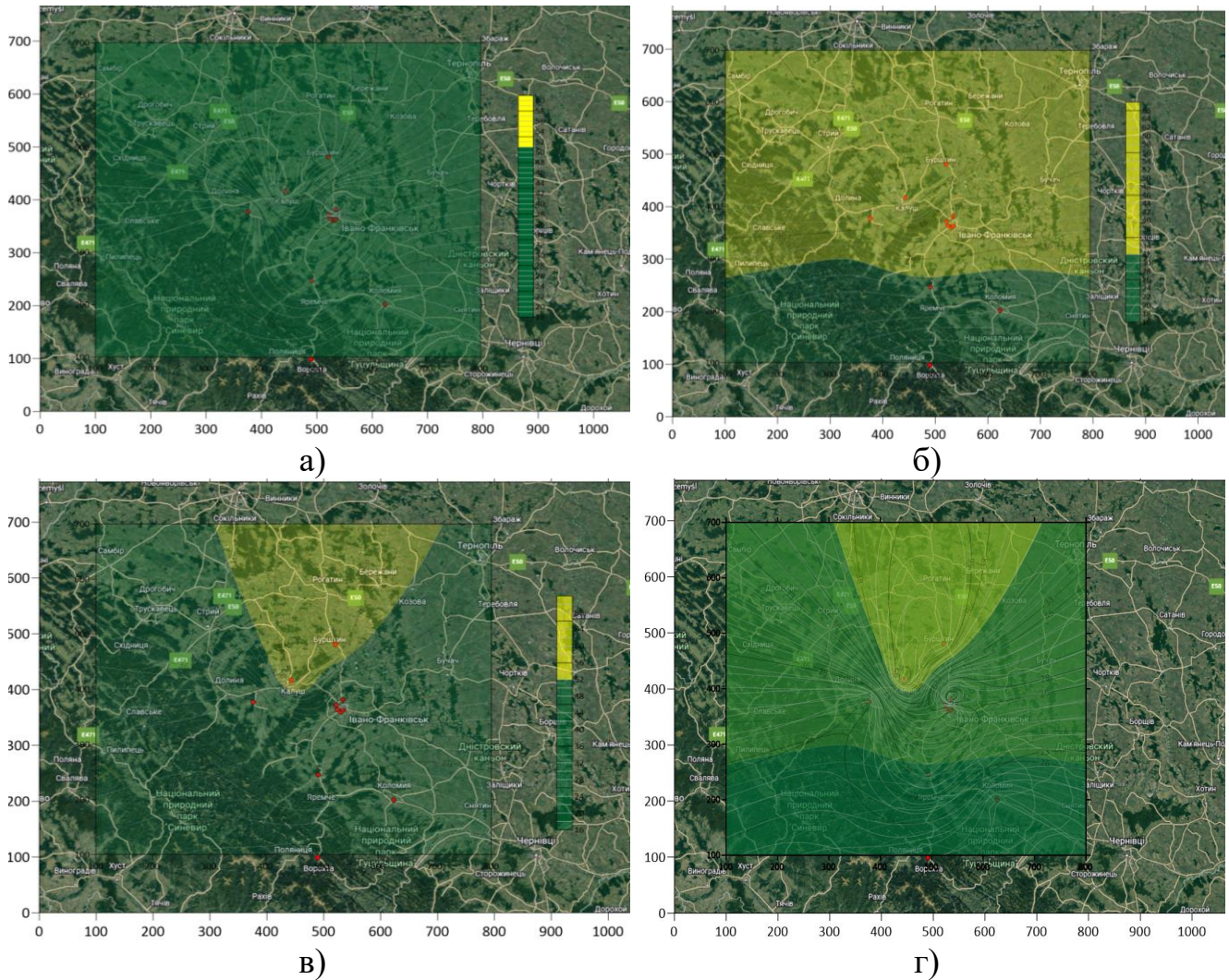
Рисунок 1 – Картограма оцінки якості атмосферного повітря: а) PM2.5; б) PM10; в) AQI; г) комплексне накладання
