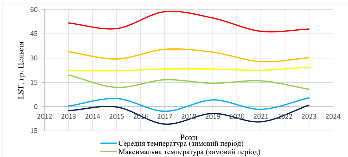
Рисунок 1 – Багаторічна динаміка показників LST у м. Маріуполь
