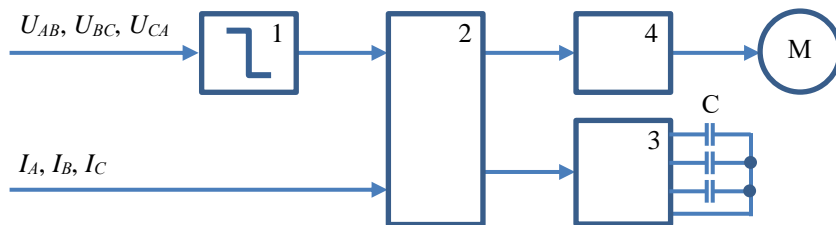
Рисунок 1. Структурна схема пристрою полегшення роботи електродвигуна
