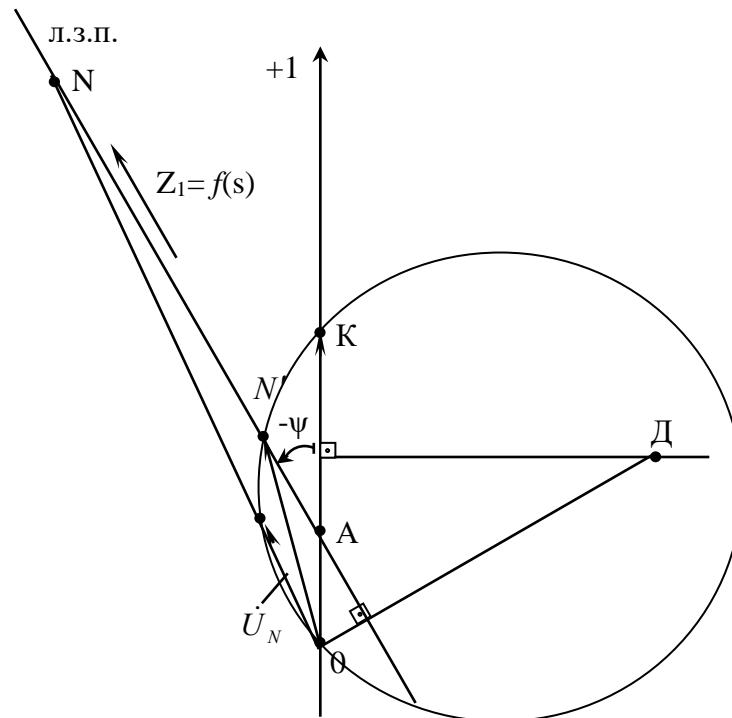
Рис. 1 – Круговая діаграма для дослідження напруги зміщення нейтралі
