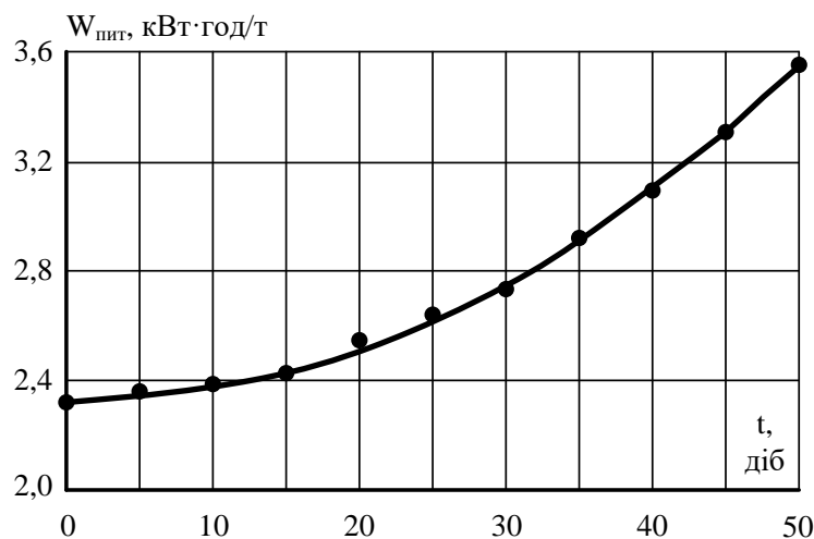
Рисунок 1 – Залежність питомої витрати електроенергії на подрібнення від часу роботи вальцевого станка (для 1 драної системи)
