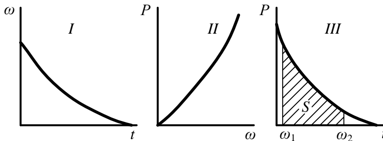
I – крива вибігу; II – втрати холостого ходу; III – крива втрат в досліді вибігу Рисунок 2 – Графіки до розрахунку моменту інерції за методом площин
