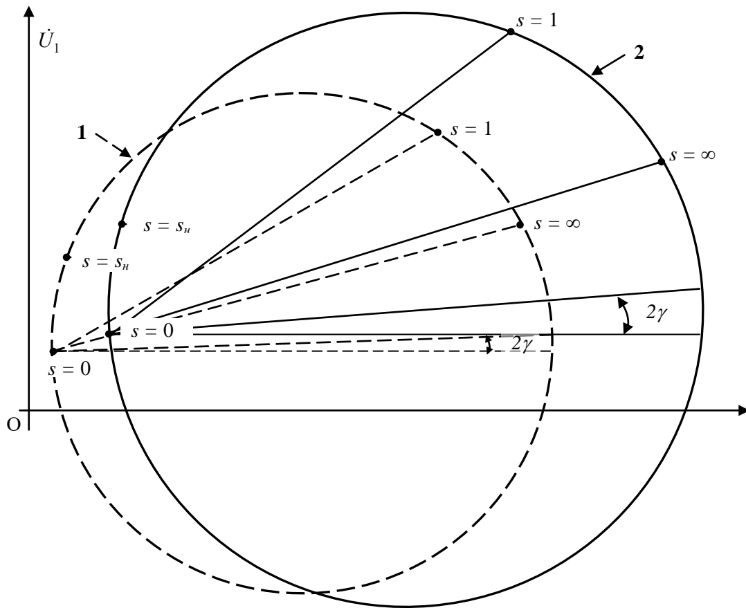
1 – базова (номінальна) кругова діаграма; 2 - кругова діаграма, побудована через певний час роботи електродвигуна.
