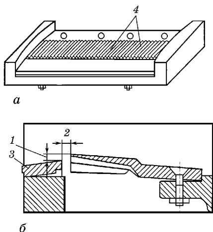
Рис. 1.38. Рама з ножами:
