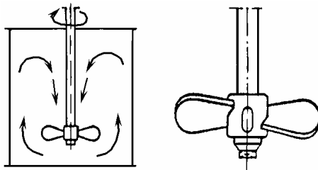
Рис. 1.54. Пропелерна мішалка
