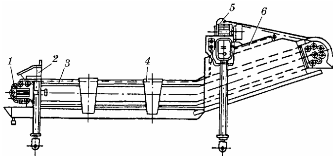
Рис. 1.24. Інспектувальний роликів конвеєр А9-КТ2-0
