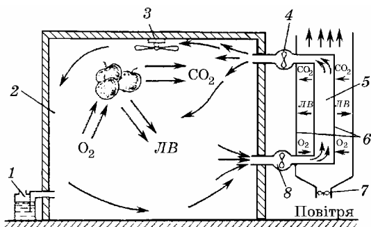
Рис. 4.13. Повітрообмін у камері для зберігання плодів у регульованому газовому середовищі, обладнаний газообмінним-дифузором фірми «Rhone Poulenc»
