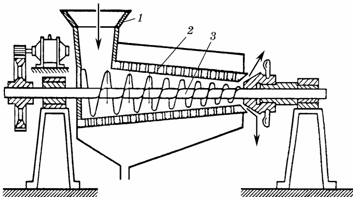
Рис. 1.71. Гвинтовий прес для відтискання олії і томатного соку
