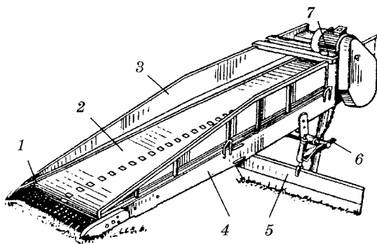
Рис. 4.16. Конвеєр-підбирач ТПК-30
