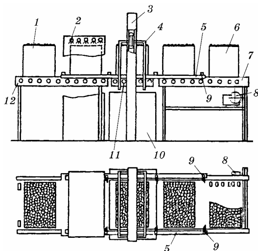
Рис. 4.22. Установка УЗП-10А
