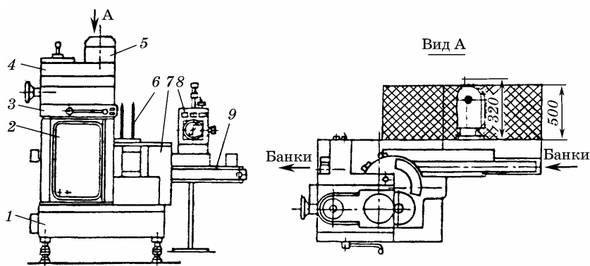
Рис. 1.110. Автомат Б4-КУТ-1
