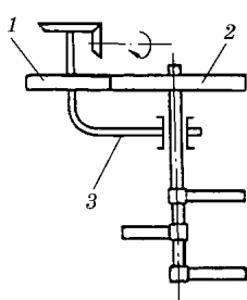
Рис. 1.53. Планетарна мішалка:
