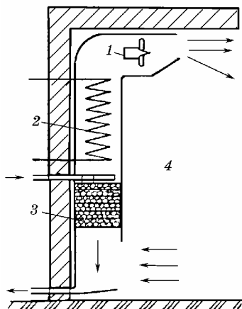
Рис. 4.3. Повітроохолоджувач:
