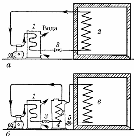
Рис. 4.2. Схема безпосереднього (а) і розсільного (б) охолодження камер зберігання продукції:
