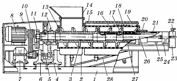
Рис. 1.74. Гвинтовий прес ВПО-20А
