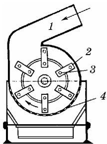
Рис. 1.43. Молоткова дробарка:
