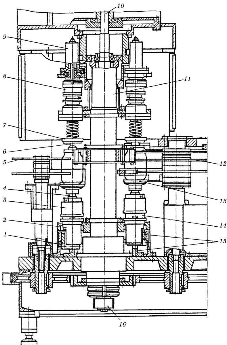
Рис. 1.111. Закупоривающий ротор автомата Б4-КУТ-2
