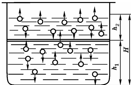
Рис. 1.27. Принципова схема дії гідравлічного сортувальника
