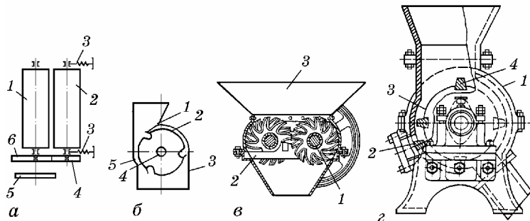
Рис. 1.41. Схеми дробарок
