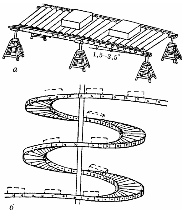
Рис. 1.6. Гравітаційний конвеєр
