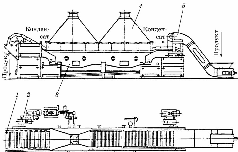
Рис. 2.11. Пароолійна піч АПМП-1
