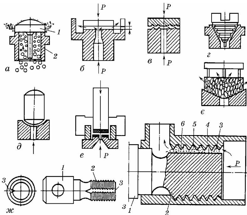
Рис. 1.47. Конструкції різних гомогенізувальних органів
