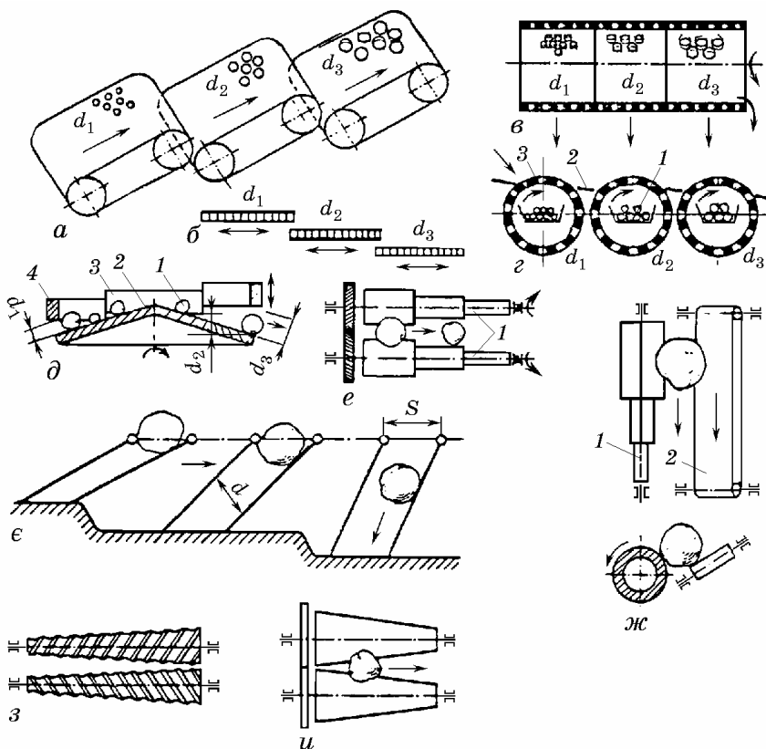
Рис. 1.28. Калібрувальні пристрої
