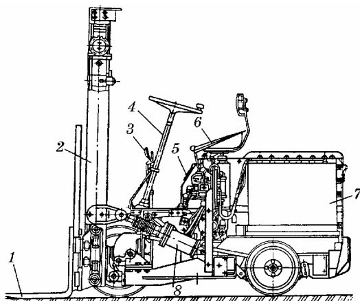
Рис. 4.18. Електронавантажувач 4004А
