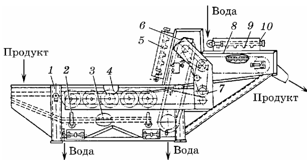
Рис. 1.15. Щіткова мийна машина Т1-КУМ-3
