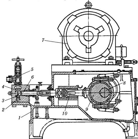
Рис. 1.48. Гомогенізатор ОГБ-5
