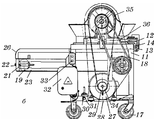
Рис. 1.40. Машина овочерізальна МШ-10000: а — загальний вигляд; б — конструкція
