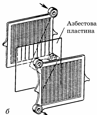
Рис. 1.87. Фільтр-прес:
