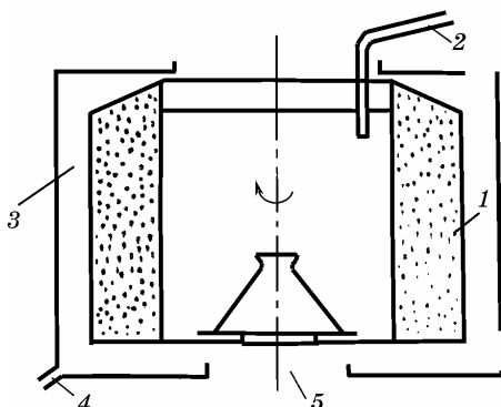
Рис. 1.81. Схема відстійної центрифуги періодичної дії:
