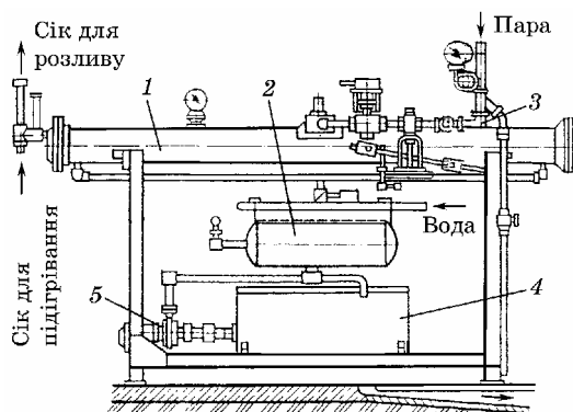
Рис. 2.7. Підігрівач КТП-2
