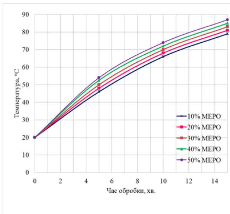
Рис. 3. Залежність температури нагрівання суміші дизельного палива і МЕРО від часу обробки
