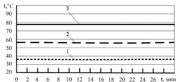
Рис. 7. Значения температуры наддувочного воздуха при работе дизеля ЯМЗ 8424 на режиме n = 1000 \text{ мин}^{-1} и N_e = 2 \text{ кВт} :
