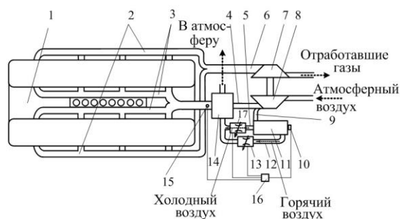
Рис. 1. Принципиальная схема системы стабилизации температуры наддувочного воздуха при работе двигателя на различных режимах с использованием вихревой трубы:
