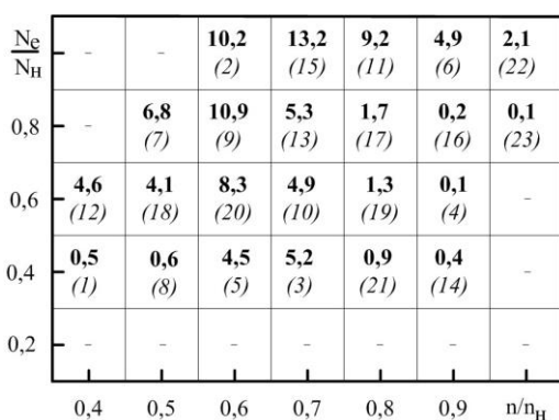
Рис. 4. Режимы работы двигателя грузового автомобиля в условиях городской эксплуатации
