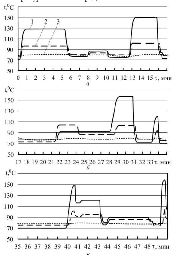
Рис. 6. Изменение температуры наддувочного воздуха при работе дизеля ЯМЗ 8424 в одном из испытательных циклов:
