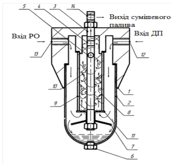
Рис. 4. Змішувач-фільтр мінерального палива і рослинної олії
