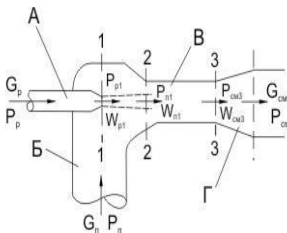
Рис. 5. Принципова схема струминного змішувача: А – робоче сопло; Б – приймальна камера; В – змішувальна камера; Р – дифузор; G - масова витрата, кг/с; P – тиск, Па; W – швидкість потоку рідини, м/с
