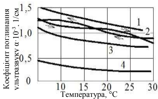
Рис. 1. Залежність коефіцієнта поглинання молока від температури:
