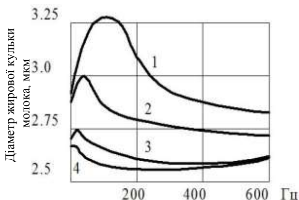
Рис. 1. Зміна середнього діаметру жирової кульки молока при дії на неї коливальних хвиль протягом 1хв.:
