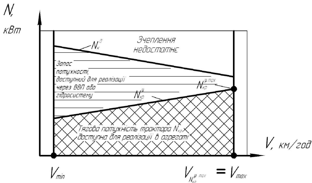
Рисунок 4 – Графік залежності тягової потужності N_{кр} від швидкості руху V в зоні недостатнього зчеплення рушія трактора із ґрунтом
