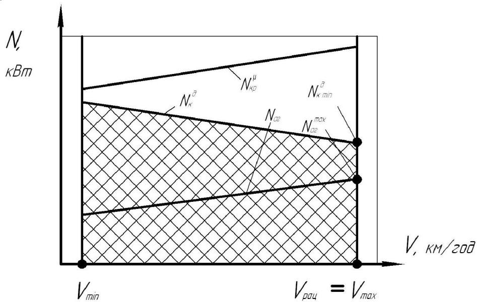
Рисунок 7 – Визначення раціональної швидкості руху агрегату в умовах достатнього зчеплення при N_{ар}^{max} \leq N_{к min}^{\mu}
