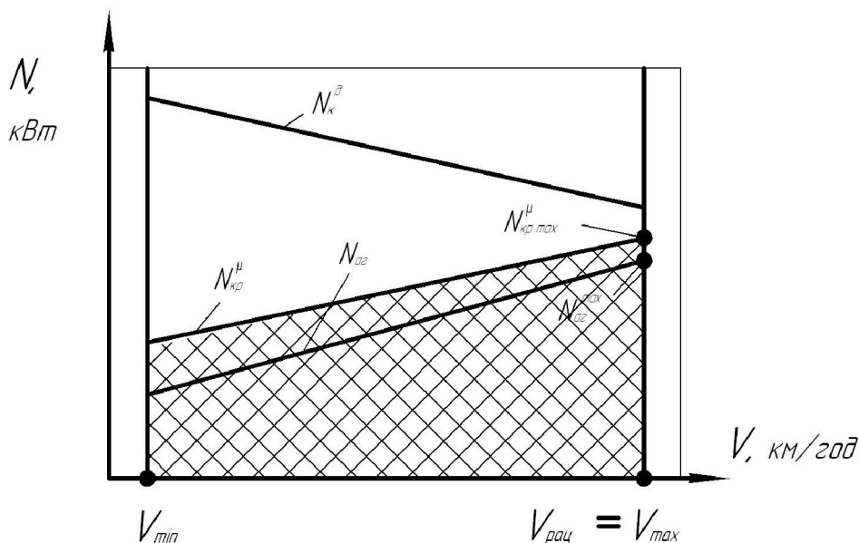
Рисунок 9 – Визначення раціональної швидкості руху агрегату в умовах недостатнього зчеплення при N_{ар}^{max} \leq N_{кр max}^{\mu}
