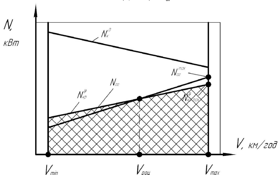
Рисунок 8 – Визначення раціональної швидкості руху агрегату в умовах недостатнього зчеплення при N_{ар}^{max} > N_{кр max}^{\mu}
