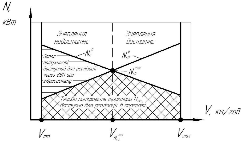
Рисунок 1 – Графік зміни корисної потужності N_k^д двигуна і тягової потужності N_k^т трактора в робочому діапазоні швидкостей руху
