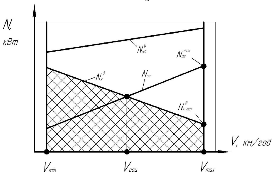
Рисунок 6 – Визначення раціональної швидкості руху агрегату в умовах достатнього зчеплення при N_{ar}^{max} > N_{кр}^D
