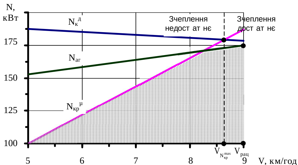
Рисунок 10 – Приклад визначення раціональної швидкості руху агрегату в умовах, якщо V_{N_{кр}^{max}} входить в інтервал агротехнічно-допустимої швидкості руху
