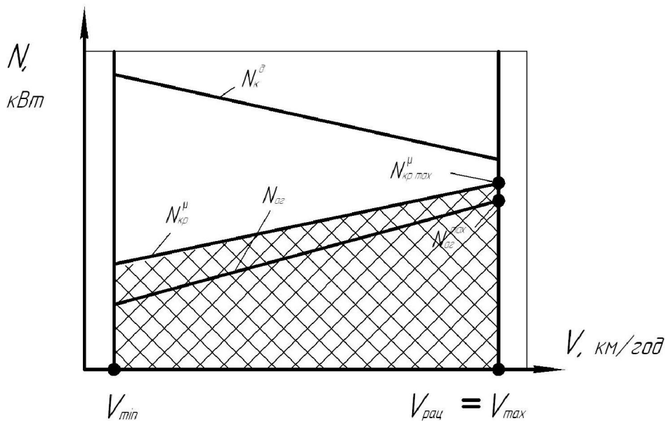
Рисунок 9 – Визначення раціональної швидкості руху агрегату в умовах недостатнього зчеплення при N_{\text{ар}}^{\text{max}} \leq N_{\text{кр max}}^{\mu}
