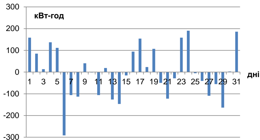
Рисунок 16 - Середньодобові небаланси енергії (добова циклічність)
