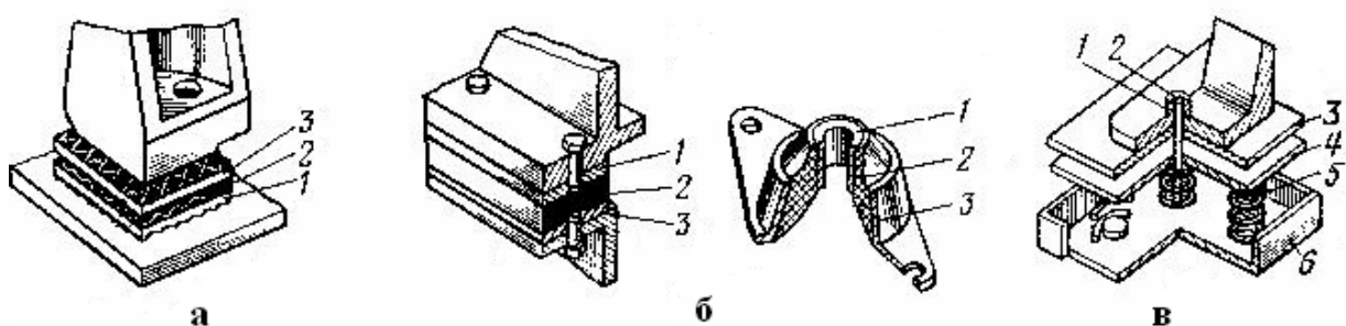
Рис. 6 - Віброзахисні пристрої: а- установка машин на пружних підкладках; 1,3 - вібростійкі підкладки; 2 - гума вулканізації; б - тришарові підкладки; 1,3 - металеві деталі; (кільця, пластини); 2 - вулканізована гума; у - пружинні амортизації: 1 - гвинт з правим і лівим різьбленням; 2 - гайка; 3,4 - пластини; 5 - пружини; 6 - підстава.
