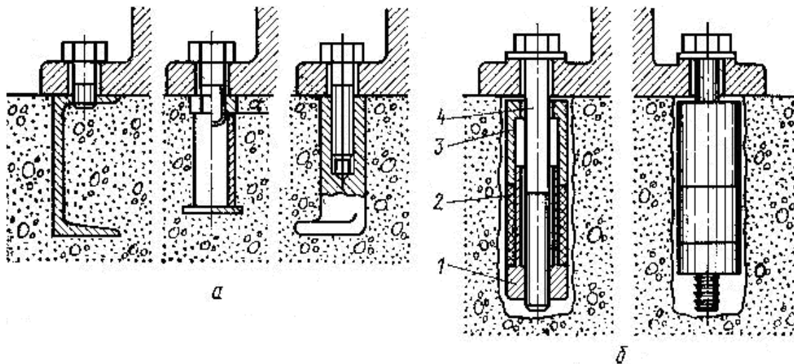
Рис. 5 - Нові види кріплень: а - фундаментні гайки; б - розтиска гумова втулка; 1 - хвостова частина; 2 - гумова втулка; 3 - обтискова втулка; 4 - болт.
