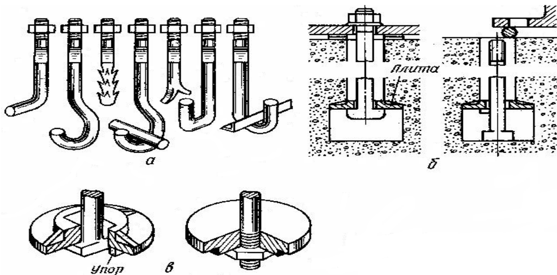
Рис. 4. Фундаментні болти: а - заливний; б - фундаментний; в - варіанти кріплення нижнього кінця фундаментного болта.
