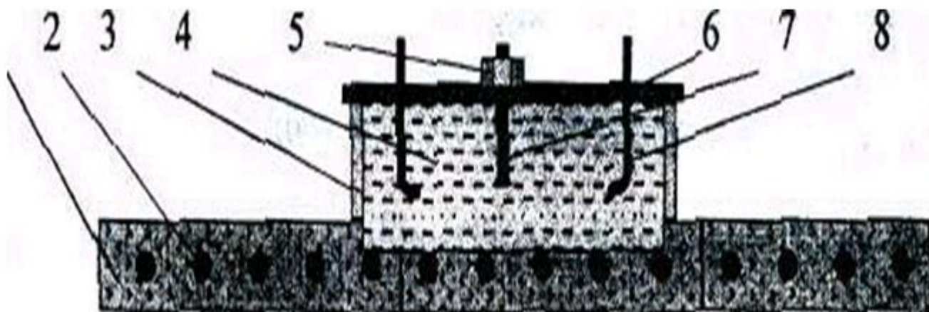
Рис. 1 Фундаментний майданчик на перекритті
