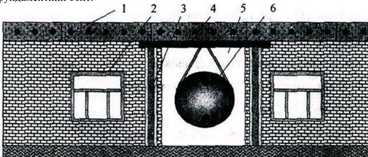
Рис. 2 Тимчасова опора в отворі несучої стіни: 1 - плита перекриття; 2 - вікно; 3 - опорна стійка; 4 - балка; 5 - отвір в стіні; 6 - технологічне обладнання, що подається в цех
