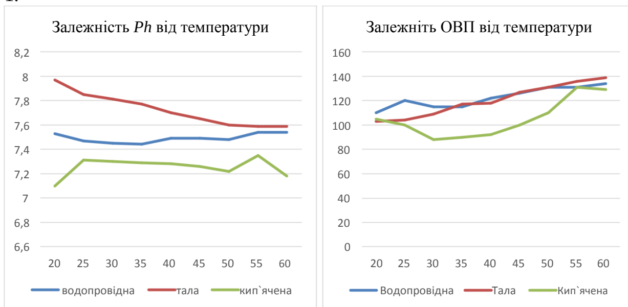
Рис. 1. Графіки залежностей ОВП і рН води від температури
