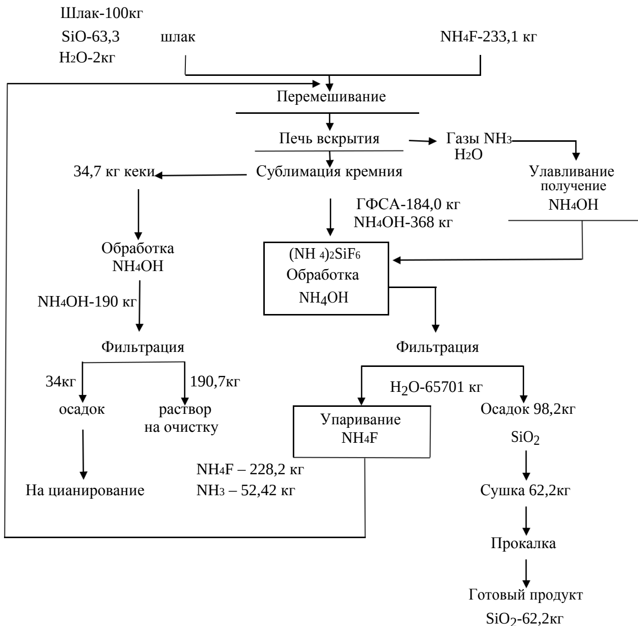
Рис. 1. Материальный баланс кремния по технологической схеме
