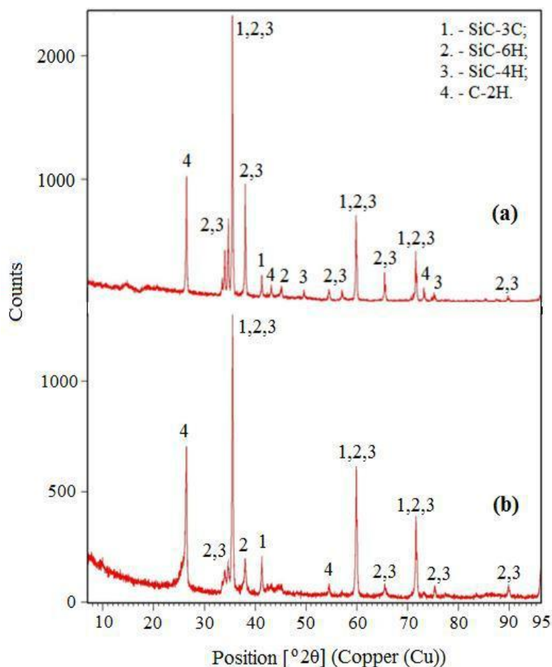
Рис. 1. Рентгенограмма синтеза порошков карбида кремния из микрокремнезема, полученных при использовании: а) нефтяного кокса; технического углерода (сажи)
