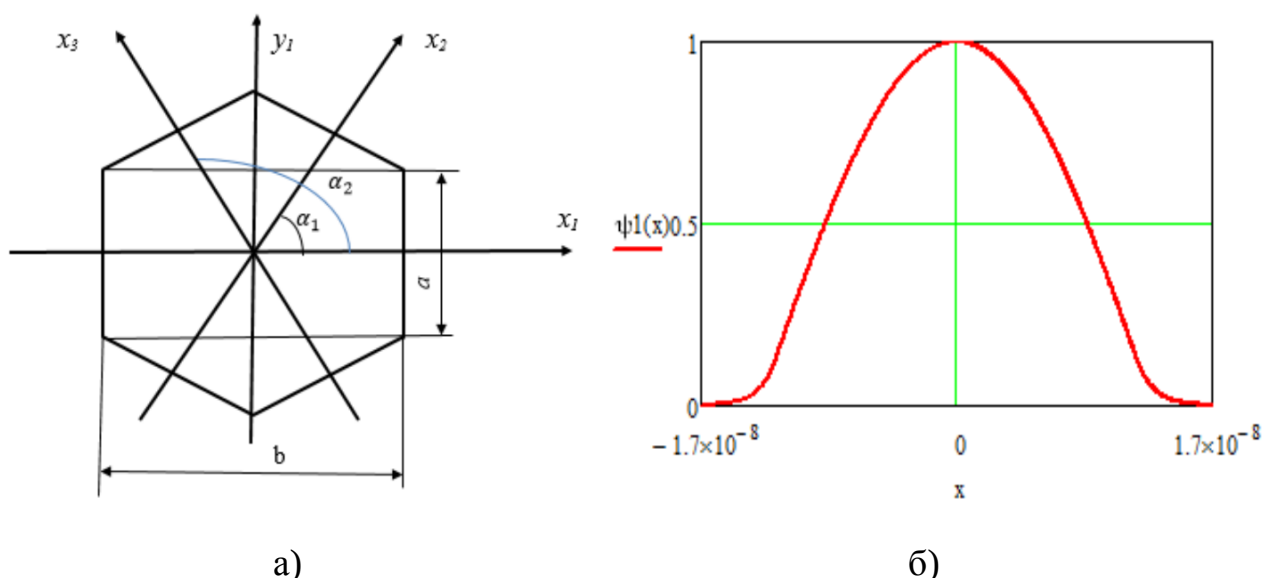
Рис. 1. Призматична квантова точка: а) переріз квантової точки: a – ширина грані, b – висота; б) графік парної хвильової функції
