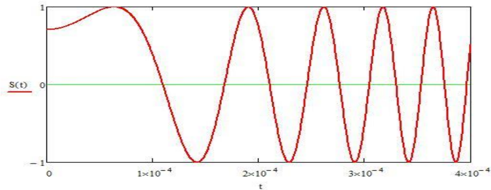
Рис. 1. Вид доплерівського сигналу з фотоприймача інтерферометра Майкельсона при \lambda = 632.8 мкм
