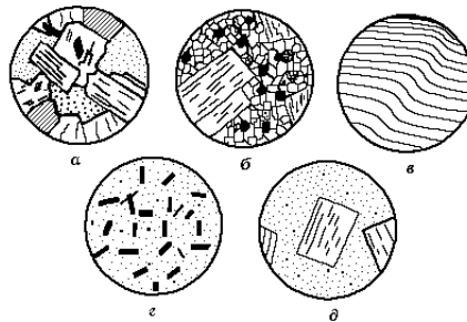
Рис. 1 Структури магматичних порід (під мікроскопом): а – повно- кристалічна, б – порфіроподібна, в – флюїдальна, з – приховано кристалічна, д - порфірова
