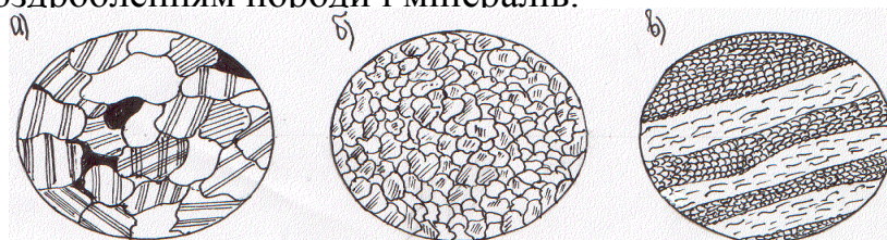
Рис.4. Структури метаморфічних порід а) - мармур; б) – кварцит; в) - гнейс
