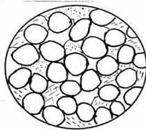
Рис. 2 Структура уламкових осадових порід
