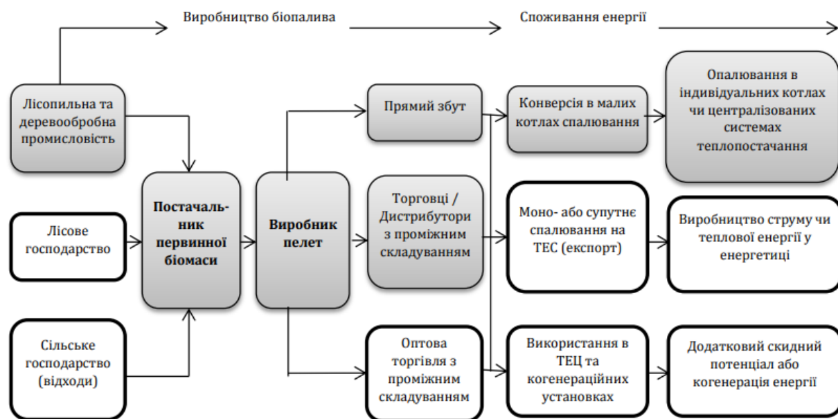
Рис. 2. Ланцюжок процесів виробництва, збуту та кінцевого використання пелет.
