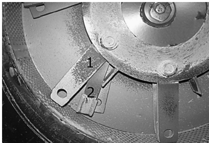
1 – серійні, 2 – експериментальні зі модульними пластинами – вставками з X13M2-Cr_3C_2-B_4C
