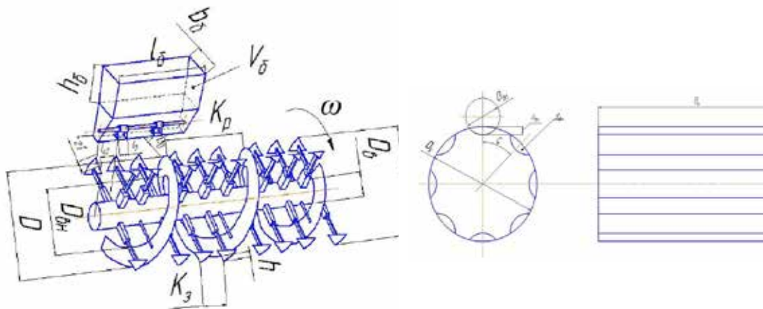
а) навантажувач-змішувач
