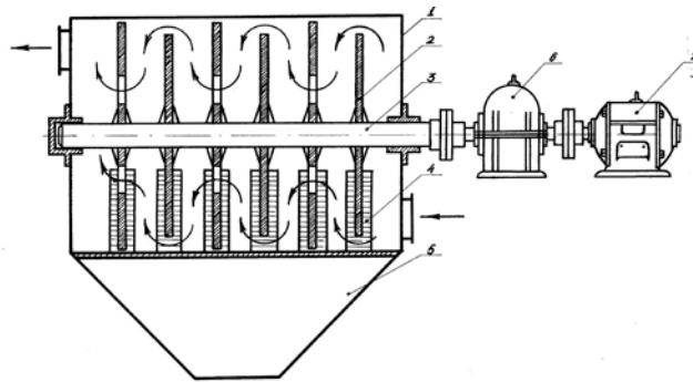
1 - корпус, 2 - диски-електроди, 3 - вал, 4 - щітки, 5 - бункер для пилу, 6 - редуктор, 7- електродвигун.
