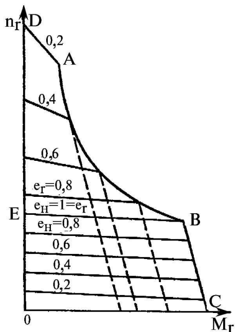
Рис. 1 Навантажувальні характеристики регульованого гідроприводу
