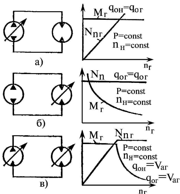
Рис.2 Варіанти об'ємного регулювання гідроприводу: а - регулювання насосом; б - регулювання гідромотором; в - регулювання насосом і гідромотором
