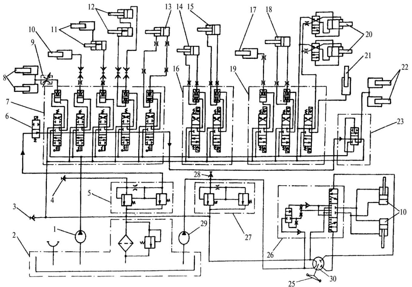
Рис. 10 Схема принципова основної гідросистеми та гідросистеми рульового керування комбайну «Дон – 1500».
