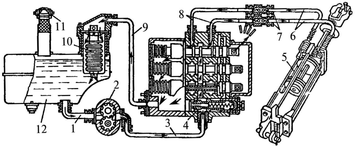
Рис. 5 Схема роздільно агрегатної навісної гідросистеми трактора: 1,3,6,8 і 9 – гідролінії; 2 – насос; 4 – гідророзподільник; 5 – гідроциліндр; 7 – запорні клапани; 10 і 11 – кондиціонери робочої рідини; 12 – робоча рідина.
