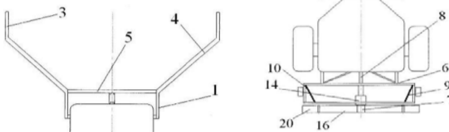
Рис. 2. Розкидачі добрив із куп передня і задня частина агрегату.
