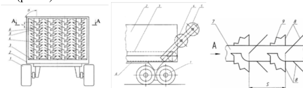
Рис. 1. Розкидачі добрив
