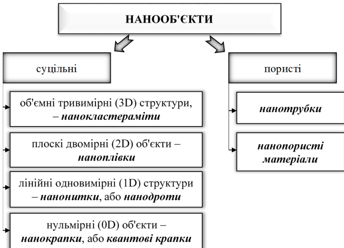
Рис. 1 –Класифікація нанооб'єктів
