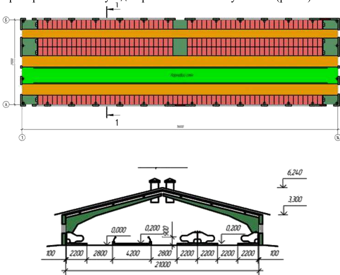
Рис. 2. Сема реконструкції (ТП801-2-49.85) корівника на 200 голів (варіант ІІ)
