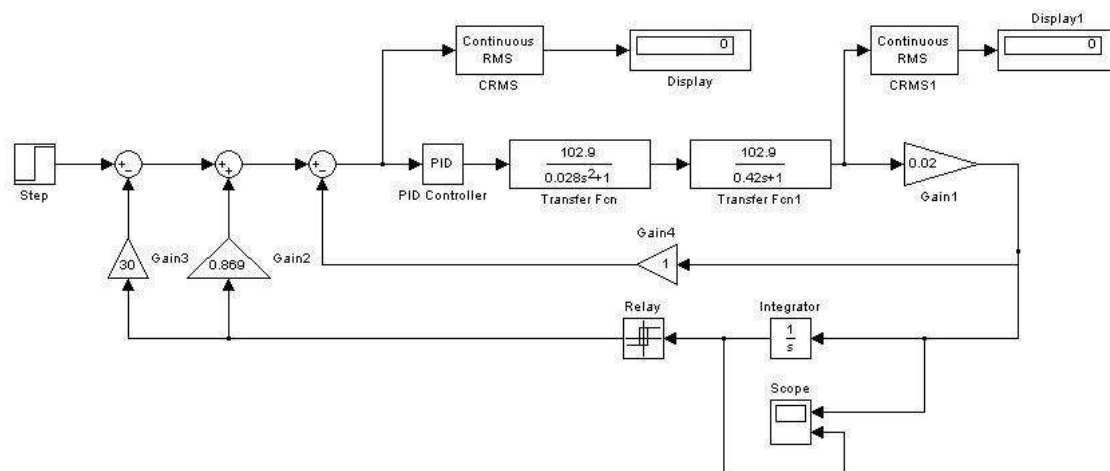
Рис. 3. Компьютерная модель регулирования уровня кислотности сырного зерна
