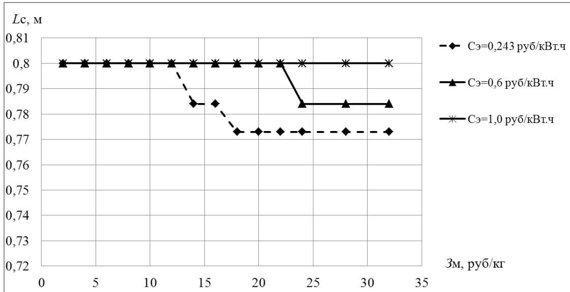
Рис. 2. Залежності L_c = f(З_M) для трансформатора типа ТМГ-100/10 со схемой соединения обмоток «звезда-двойной зигзаг с нулевым проводом»
