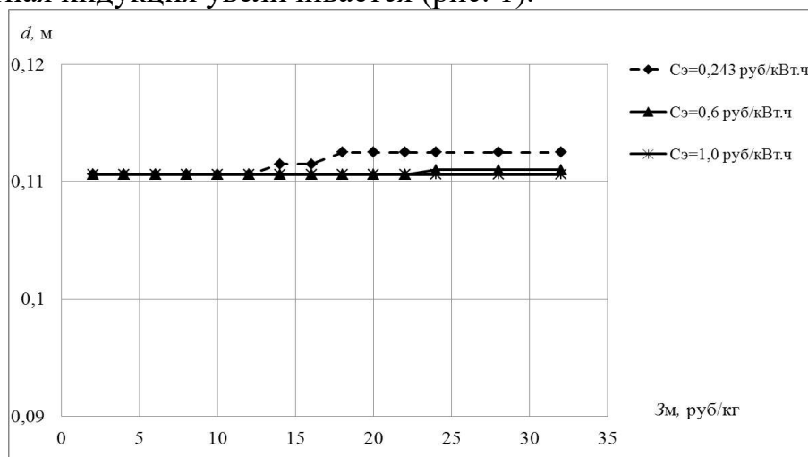
Рис. 1. Залежності d = f(Z_M) для трансформатора типа ТМГ-100/10 со схемой соединения обмоток «звезда-двойной зигзаг с нулевым проводом»
