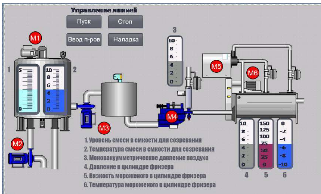
Рис. 1. Главный экран панели оператора
