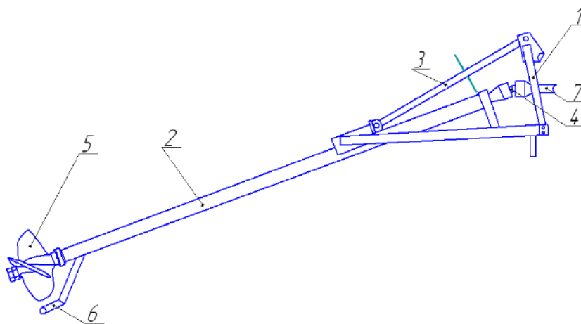
1-навеска; 2-рама; 3-талреп; 4-вал; 5-винт; 6-упор; 7-карданный вал
