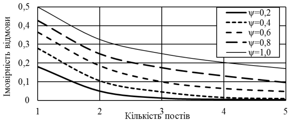
Рис. 4. Зміна імовірності відмови в обслуговуванні клієнтів в залежності від кількості постів ( n ) при різних коефіцієнтах завантаження ( \psi ) при відсутності черги ( m=0 ) та повної взаємодопомози між виконавцями
