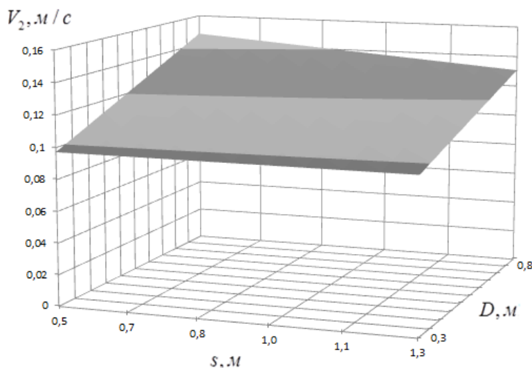
Рис. 1. Зависимость скорости движения навозной массы по каналу от диаметра мешалки и высоты навозной массы
