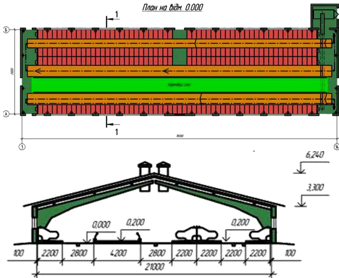
Рис. 1. Схема реконструкції корівника (ТП 801-2-49.85) на 200 голів (варіант І)
