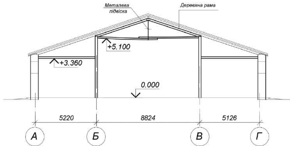
Рис. 2. Поперечний переріз будівлі зерноскладу №2
