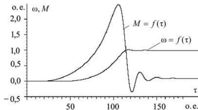
Рис. 2. Графіки перехідних процесів швидкості та моменту при пуску асинхронного двигуна через тиристорний пусковий пристрій.
