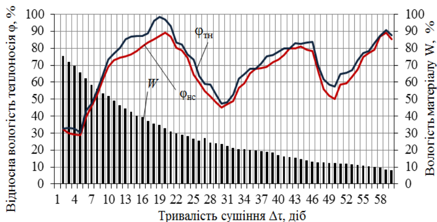
Рис. 3. Кінетичні параметри процесів вологовіддачі в геліосушарці у період з 1.06.2021 р. по 29.07.2021 р. [2]
