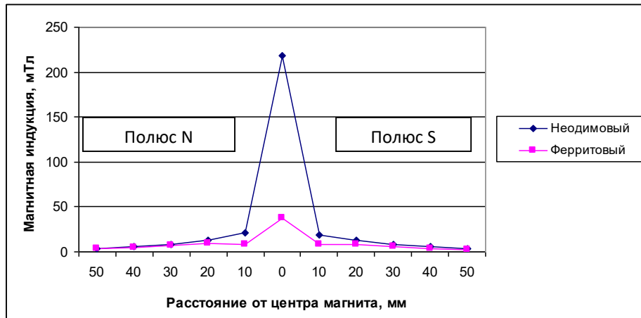
Рис. 3. Розповсюдження магнітної індукції від кільцевих магнітів без додаткових пристроїв (пристрій ІОН-3)
