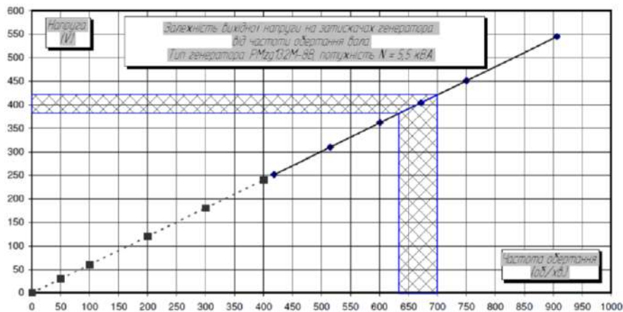
Рис. 1. Вихідна характеристика електрогенератора PMzg32M-8В потужністю 5,5 кВА зі збудженням за допомогою постійних магнітів
