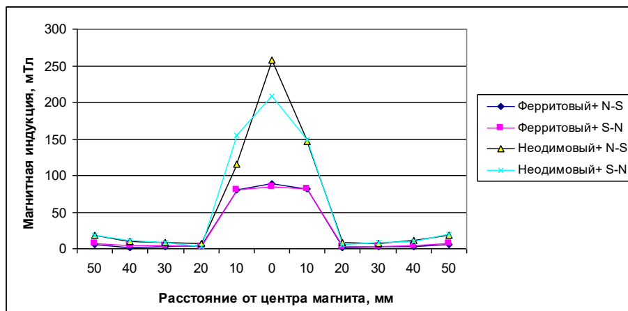
Рис. 4. Зміна магнітної індукції по осі пристрою при різній орієнтації ферритового та неодимового магнітів (пристрій ІМП-1)
