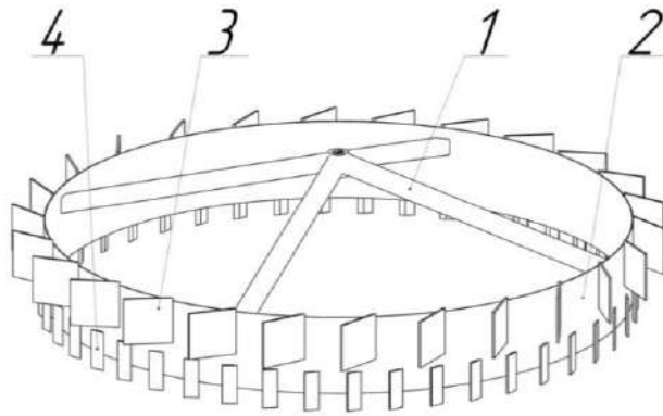
Рис. 4. Подгребающий узел
