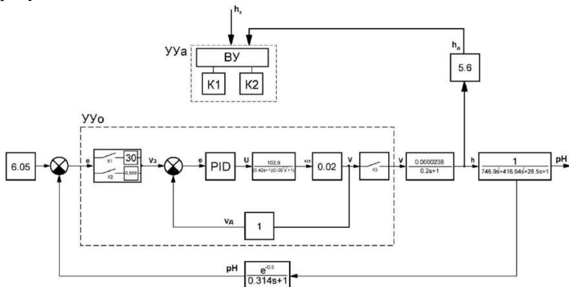
Рис. 2. Структурная схема регулирования уровня кислотности сырого зерна
