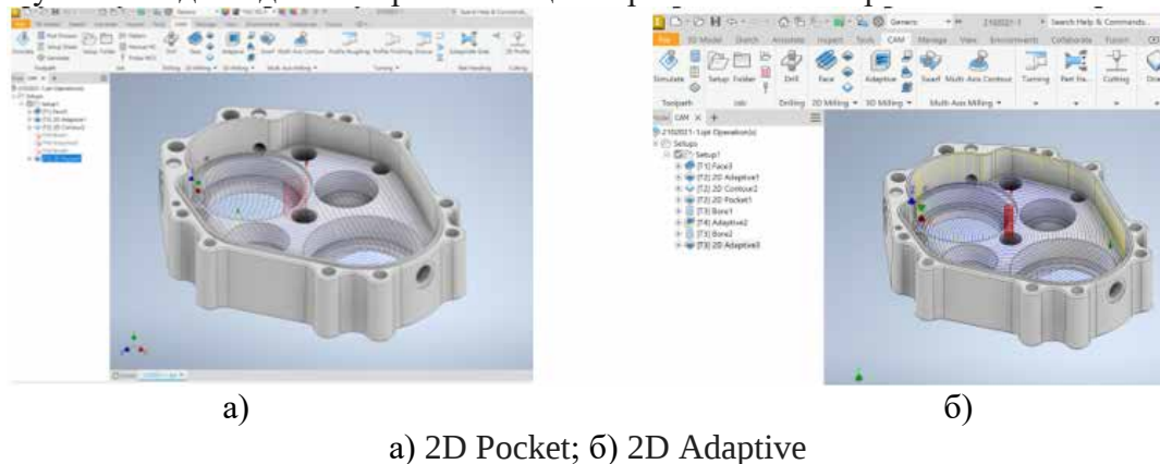
Рис. 1. Стратегії обробки внутрішньої поверхні деталі:
