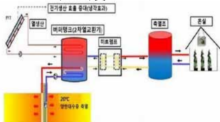
Рис. 1. Когенераційна фотоелектрична система для теплиць (Південна Корея)
