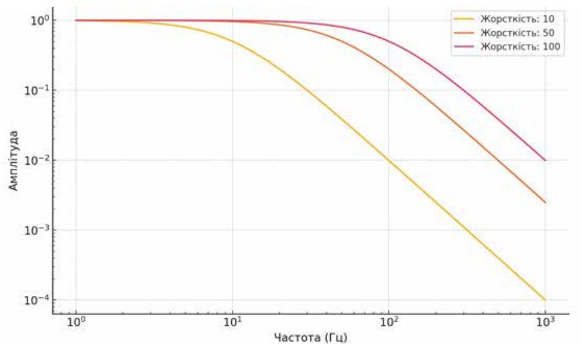
Рис. 2. Амплітудно-частотні характеристики відпрацювання копачем коливань профілю шляху з різною жорсткістю шин його коліс: 1 – 10 кН/м; 2 – 50 кН/м; 3 – 100 кН/м
