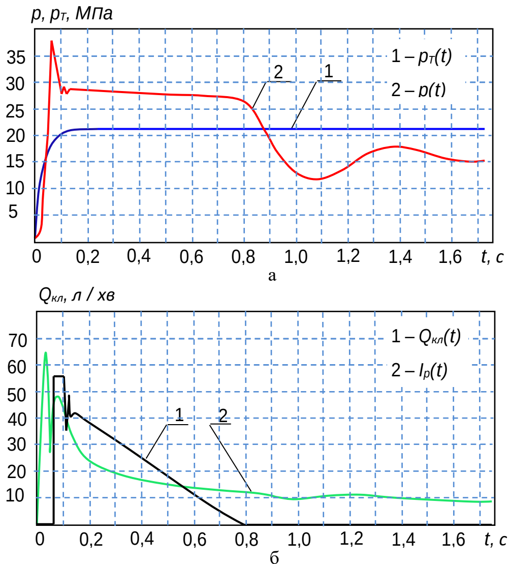
Рис. 2. Характеристика процесу розгону гідроприводу мехатронної системи при вихідних значеннях оптимізуються параметрів клапана C_x = 200 \text{ Н/см} , x_z = 0,53 \text{ см} , x_0 = 0,125 \text{ см} : а – зміна тиску; б – зміна критерію оптимізації по тиску
