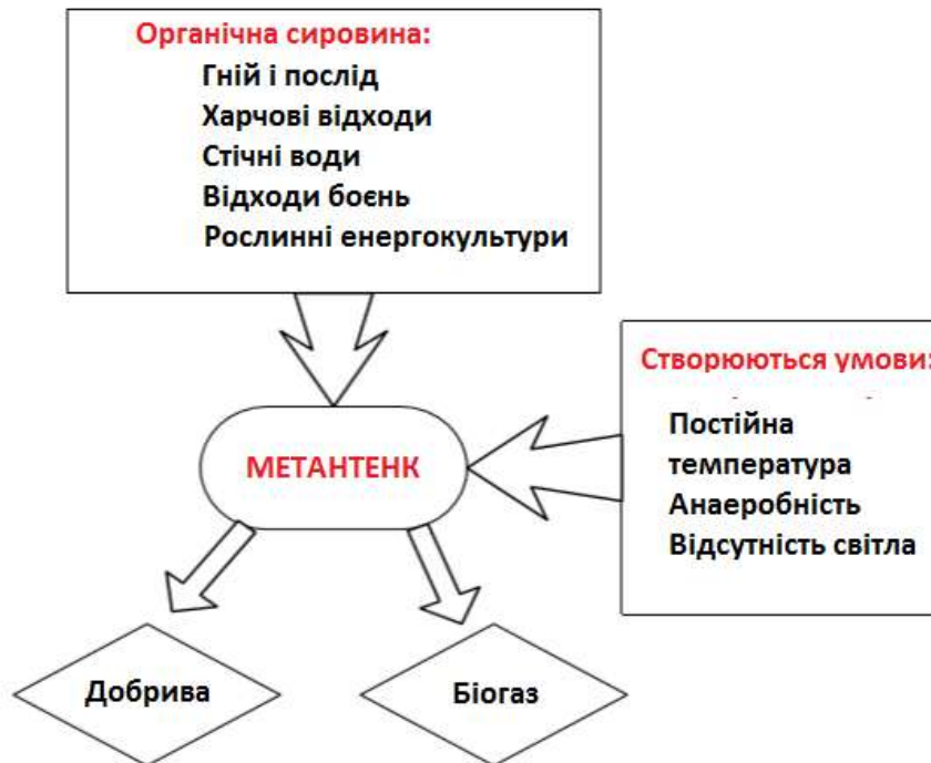
Рис. 2. Спрощена схема процесу анаеробного зброджування
