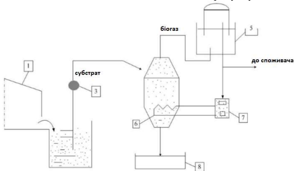
Рис.1. Принципова блок-схема біогазових установок:
