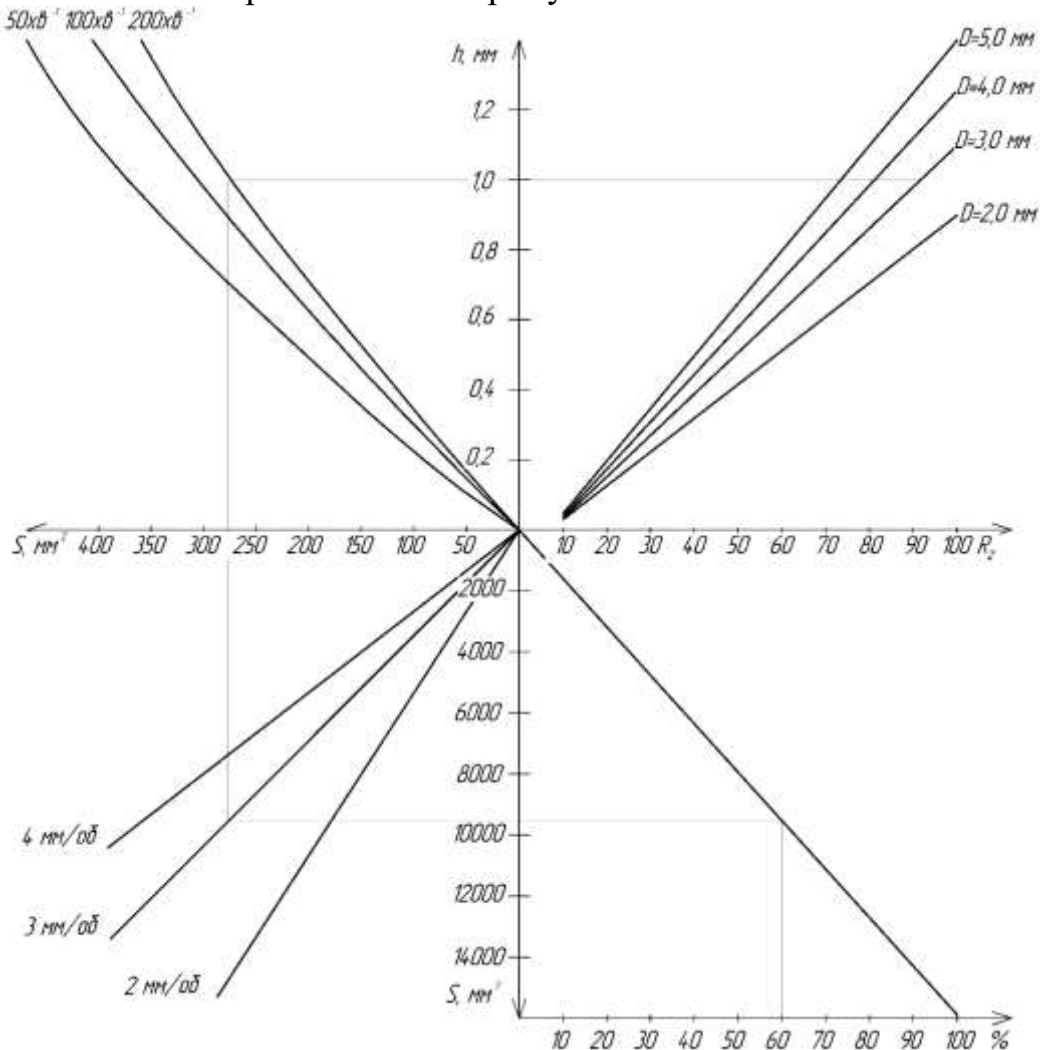
Рисунок 1 – Номограма для визначення режимів вібронакатування втулки
