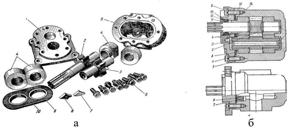
Рисунок 1.1 – Будова насосу НШ-У:
