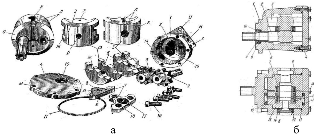
Рисунок 1.2 – Будова насосу НШ – К:
