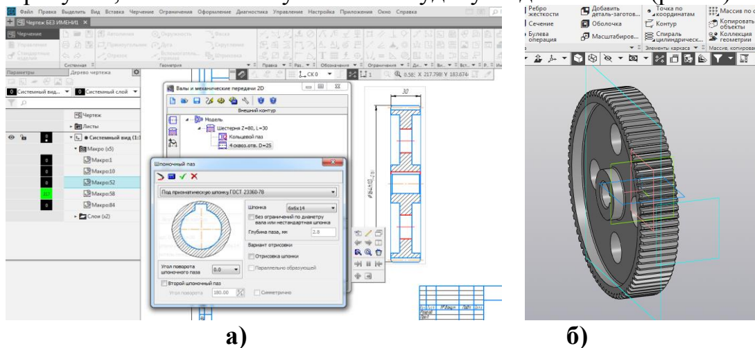
Рис. 1. Циліндричне зубчасте колесо а) побудова креслення; б) тривимірна модель
