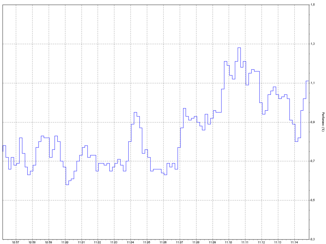
Рис. 5. График изменения уровня коэффициента несимметрии напряжения по обратной последовательности на ТП 648 «н.п. Дещенка ВРУ молочно-товарного комплекса (ввод 2)»
