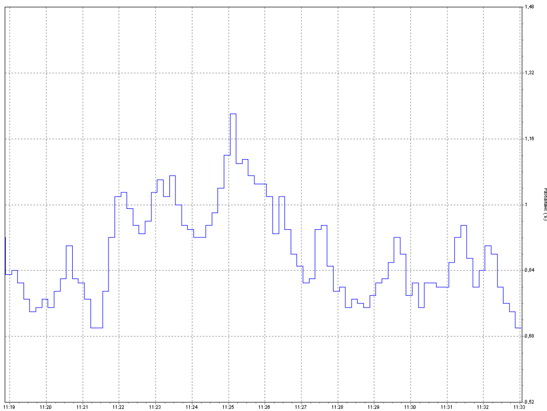
Рис. 2. График изменения коэффициента несимметрии напряжения по обратной последовательности на ТП 648 «н.п. Дещенка ВРУ молочно-товарного комплекса (ввод 1)»
