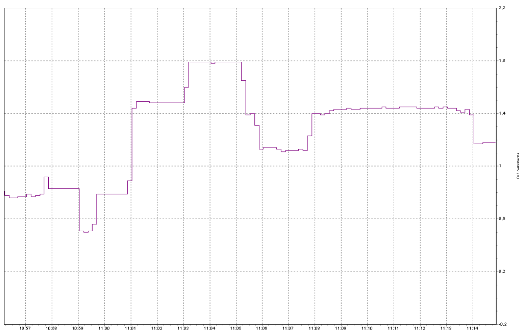
Рис. 6. График изменения коэффициента несимметрии напряжения по нулевой последовательности на ТП 648 «н.п. Дещенка ВРУ молочно-товарного комплекса (ввод 2)»
