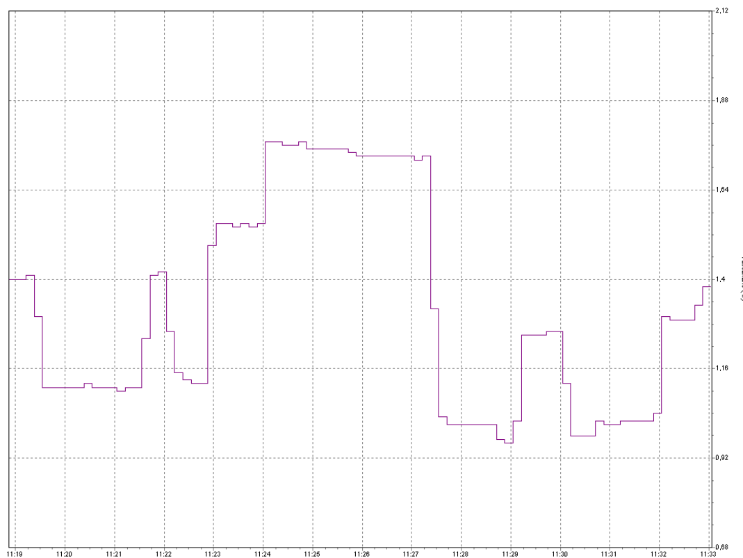
Рис. 3. График изменения коэффициента несимметрии напряжения по нулевой последовательности на ТП 648 «н.п. Дещенка ВРУ молочно-товарного комплекса (ввод 1)»
