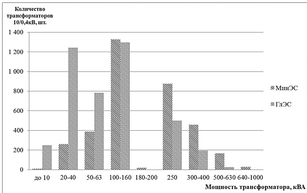
Рис. 1. Количество трансформаторов различной мощности установленных в ЭС
